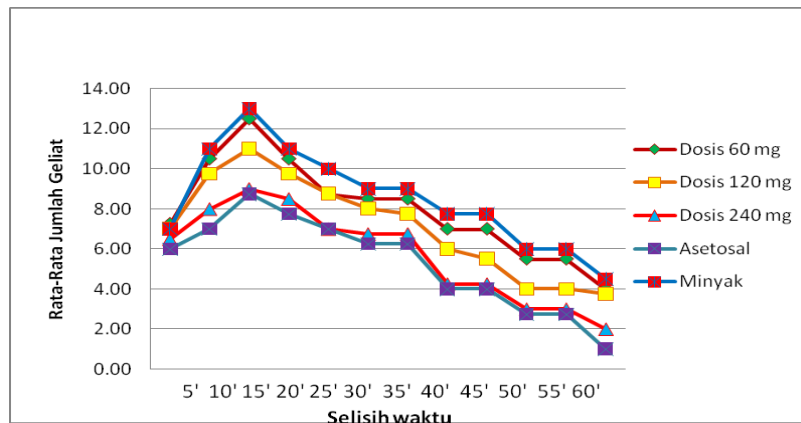
Gambar 6. Grafik Hubungan antara Waktu Percobaan dengan Geliat pada Hewan Uji Mencit pada analgetik
