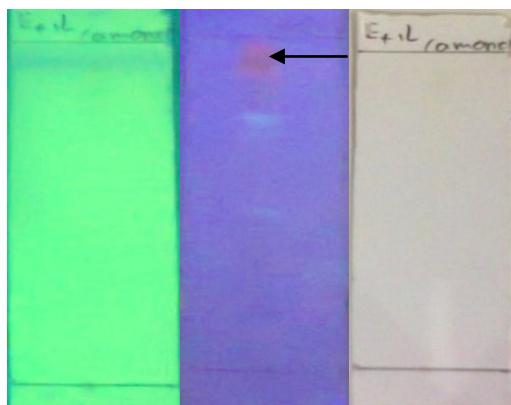
Gambar4.14 ekstrak etil asetat pada sinar UV 254nm, 366nm dan setelah diuapi amonia
