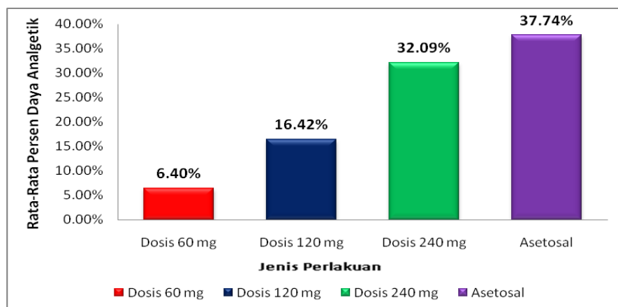
Gambar 8. Diagram Hubungan antara jenis perlakuan dengan rata-rata persen daya analgetik
